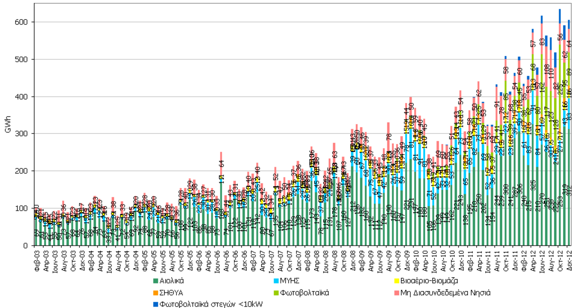
2003 – 2012 ΕΘΝΙΚΗ ΠΑΡΑΓΩΓΗ ΗΛΕΚΤΡΙΚΗΣ ΕΝΕΡΓΕΙΑΣ (GWh) ΜΟΝΑΔΩΝ ΑΠΕ & ΣΗΘΥΑ (Άρθρα 9 & 10 Ν.3468/2006) & Φ/Β ΣΤΕΓΩΝ <10kW
