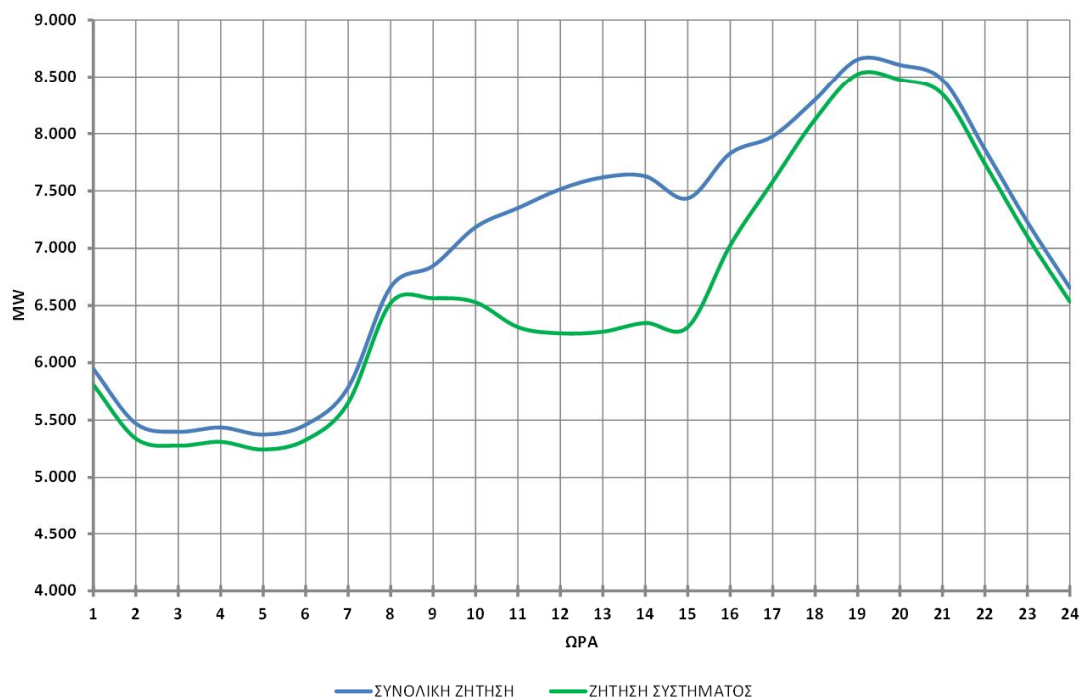
ΩΡΙΑΙΑ ΖΗΤΗΣΗ ΚΑΤΑ ΤΗΝ ΗΜΕΡΑ ΣΥΝΟΛΙΚΟΥ ΜΕΓΙΣΤΟΥ ΤΟΥ ΜΗΝΑ: 12/12/2013
