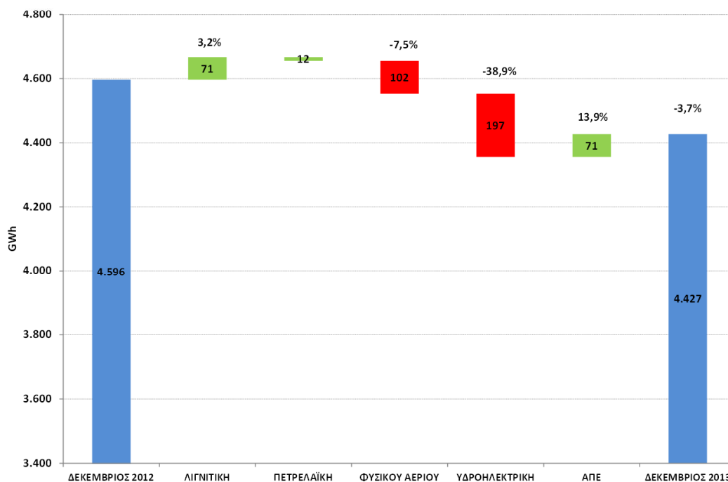
ΜΕΤΑΒΟΛΗ ΠΑΡΑΓΩΓΗΣ ΔΕΚΕΜΒΡΙΟΥ 2012 ΕΝΑΝΤΙ ΔΕΚΕΜΒΡΙΟΥ 2013 (GWh)
