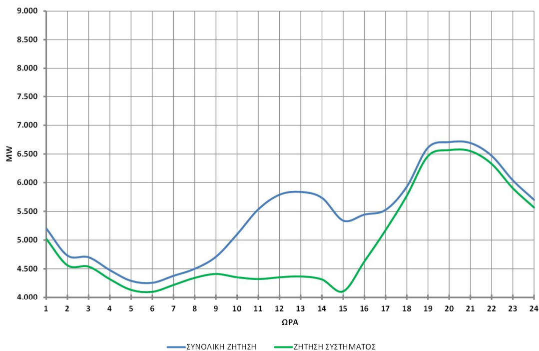
ΩΡΙΑΙΑ ΖΗΤΗΣΗ ΚΑΤΑ ΤΗΝ ΗΜΕΡΑ ΣΥΝΟΛΙΚΟΥ ΕΛΑΧΙΣΤΟΥ ΤΟΥ ΜΗΝΑ: 29/12/2013
