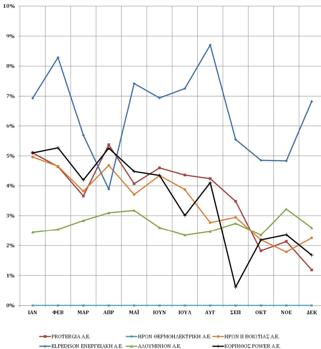
ΠΟΣΟΣΤΟ ΚΑΘΑΡΗΣ ΠΑΡΑΓΩΓΗΣ ΑΠΟ ΣΥΜΒΑΤΙΚΕΣ ΜΟΝΑΔΕΣ ΣΤΟ ΣΥΣΤΗΜΑ (ΠΛΗΝ ΔΕΗ Α.Ε.)
